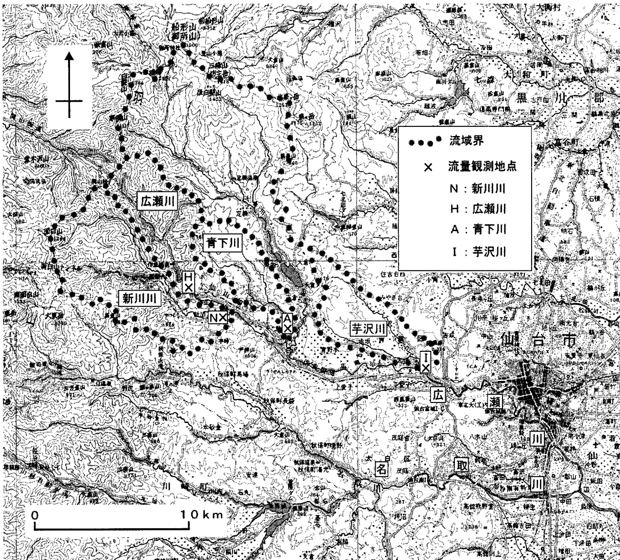
図1 広瀬川水系と研究対象流域 数値地図 200000 「日本-II」(国土地理院発行) をもとに作成
