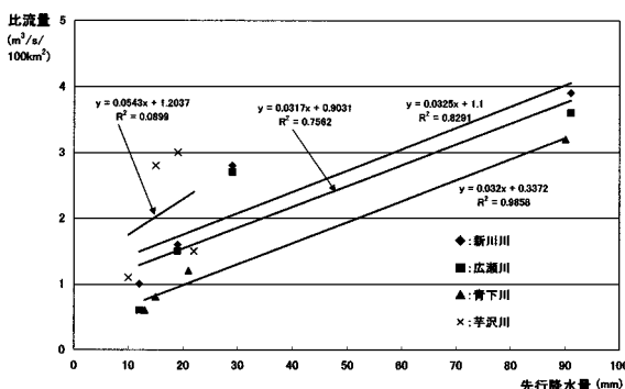
図3 先行降水量と比流量の関係
