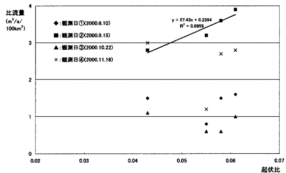
図4 各流域の起伏比と比流量の関係
