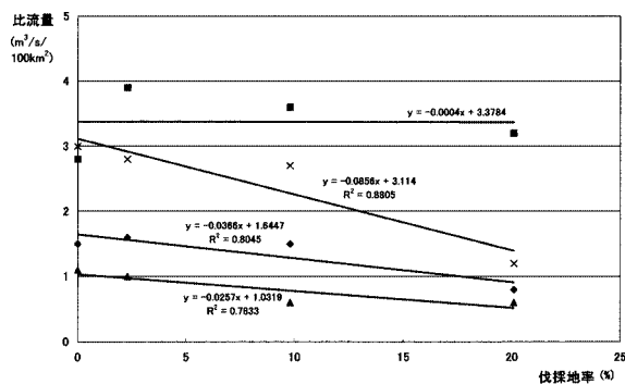
図5 各流域の伐採地率と比流量の関係 凡例は図4と同じ
